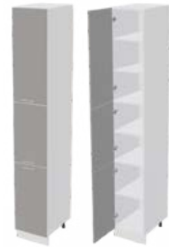
Корпус: ШПВ400 400x2320x566 (ШxВxГ) Фасад: ШПВ400 397x715x16 (ШxВxГ) - 1 шт. 397x597x16 (ШxВxГ) - 1 шт. 397x895x16 (ШxВxГ) - 1 шт.
