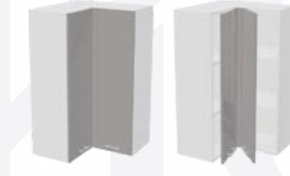
Корпус: ШВУП600x900 / 600x898x600 (ШxBxГ) Фасад: ШВУП600x900 262x895x16 (ШxBxГ) - 2 шт. 90x895x16 (ШxBxГ) - 1 шт. 34x895x16 (ШxBxГ) - 1 шт.
