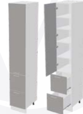
Корпус: ШПВ2Я400-1 400x2320x566 (ШxВxГ) Фасад: ШПВ2Я400-1 397x1496x16 (ШxВxГ) - 1 шт. 397x356x16 (ШxВxГ) - 2 шт.
