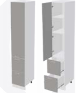
Корпус: ШП2Я400-1 400x2140x553 (ШxBxГ) Фасад: ШП2Я400-1 397x1317x16 (ШxBxГ) - 1 шт. 397x356x16 (ШxBxГ) - 2 шт.
