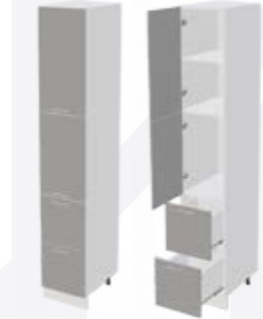
Корпус: ШП2Я400 400x2140x553 (ШxBxГ) Фасад: ШП2Я400 397x715x16 (ШxBxГ) - 1 шт. 397x597x16 (ШxBxГ) - 1 шт. 397x356x16 (ШxBxГ) - 2 шт.
