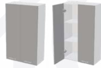
Корпус: ШВ600x900 / ШВС600x900 600x898x283 (ШxBxГ) Фасад: ШВ600x900 297x895x16 (ШxBxГ) - 2 шт.
