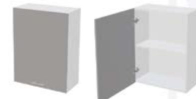
Корпус: ШВ1Д600 / ШВС1Д600 600x718x283 (ШxВxГ) Фасад: ШН1Д600 / ШНМ1Д600 / ШВ1Д600 597x715x16 (ШxВxГ) - 1 шт.
