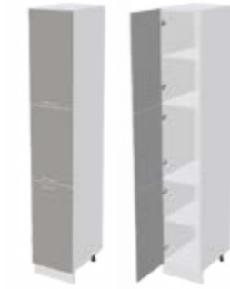
Корпус: ШП400 400x2140x553 (ШxBxГ) Фасад: ШП400 397x715x16 (ШxBxГ) - 2 шт. 397x597x16 (ШxBxГ) - 1 шт.
