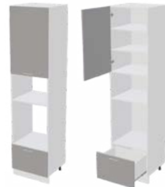
Корпус: ШПВ2Я400 400x2320x566 (ШxВxГ) Фасад: ШПВ2Я400 397x895x16 (ШxВxГ) - 1 шт. 397x597x16 (ШxВxГ) - 1 шт. 397x356x16 (ШxВxГ) - 2 шт.
