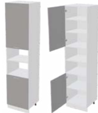
Корпус: ШПВ600 600x2320x566 (ШxВxГ) Фасад: ШПВ600 597x715x16 (ШxВxГ) - 1 шт. 597x895x16 (ШxВxГ) - 1 шт.
