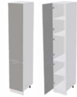
Корпус: ШП400-1 400x2140x553 (ШxBxГ) Фасад: ШП400-1 397x1317x16 (ШxBxГ) - 1 шт. 397x715x16 (ШxBxГ) - 1 шт.
