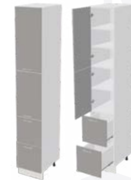
Корпус: ШПВ2Я400 400x2320x566 (ШxВxГ) Фасад: ШПВ2Я400 397x895x16 (ШxВxГ) - 1 шт. 397x597x16 (ШxВxГ) - 1 шт. 397x356x16 (ШxВxГ) - 2 шт.
