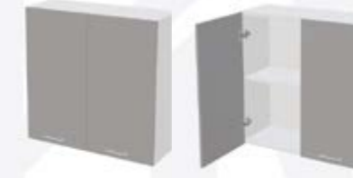
Корпус: ШВ800 / ШВС800 800x718x283 (ШxВxГ) Фасад: ШН800 / ШНМ800 / ШВ800 397x715x16 (ШxВxГ) - 2 шт.
