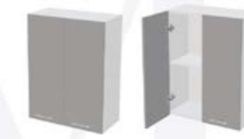
Корпус: ШВ600 / ШВС600 600x718x283 (ШxВxГ) Фасад: ШН600 / ШНМ600 / ШВ600 297x715x16 (ШxВxГ) - 2 шт.
