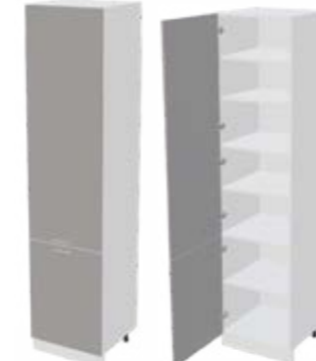
Корпус: ШПВ600-2 600x2320x566 (ШxВxГ) Фасад: ШПВ600-2 597x1496x16 (ШxВxГ) - 1 шт. 597x715x16 (ШxВxГ) - 1 шт.
